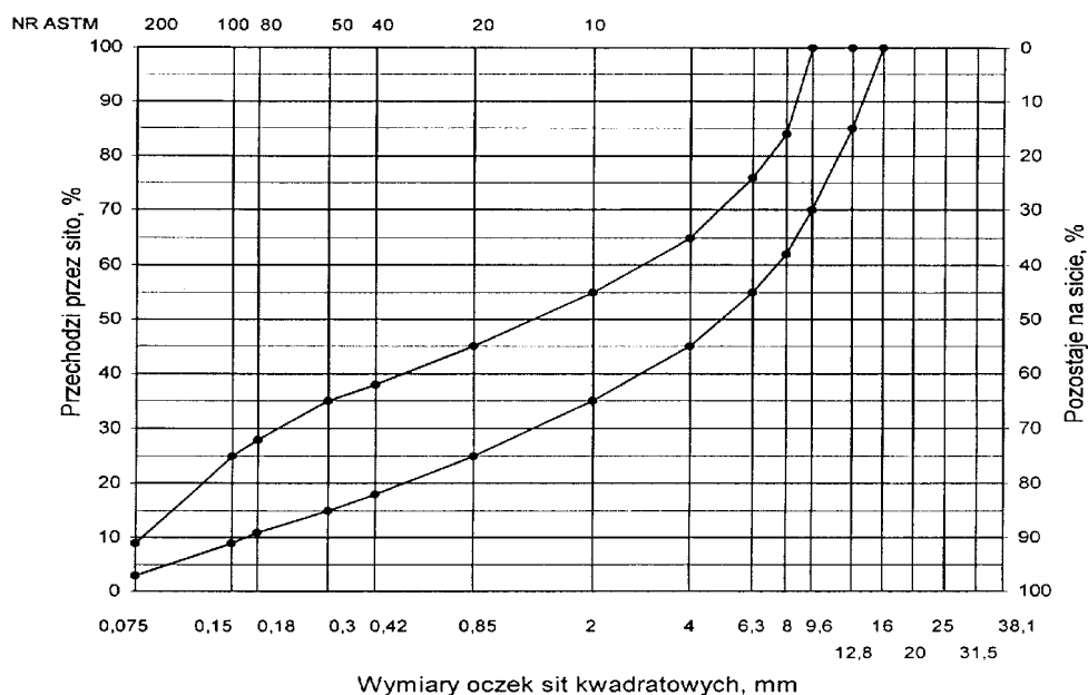
Rys. 3. Krzywe graniczne uziarnienia mieszanki mineralnej BA od 0 do 12,8 mm do warstwy wiążącej nawierzchni drogi o obciążeniu ruchem KR1 lub KR2
