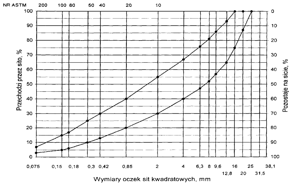
Rys. 1. Krzywe graniczne uziarnienia mieszanki mineralnej BA od 0 do 20 mm do warstwy wiążącej nawierzchni drogi o obciążeniu ruchem KR1 lub KR2
