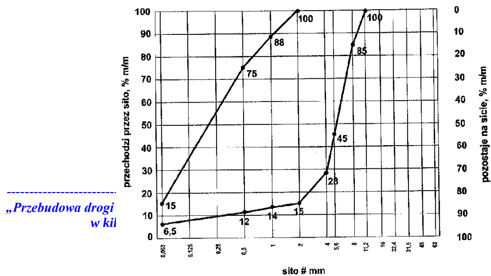
Rys. 4. Krzywe graniczne uziarnienia mieszanki mineralnej 0/11,2 mm
