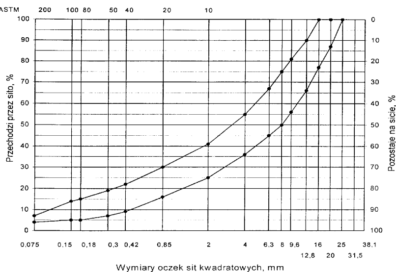
Rys. 5. Krzywe graniczne uziarnienia mieszanki mineralnej BA od 0 do 25 mm do warstwy wiążącej, wyrównawczej i wzmacniającej nawierzchni drogi o obciążeniu ruchem od KR3 do KR6
