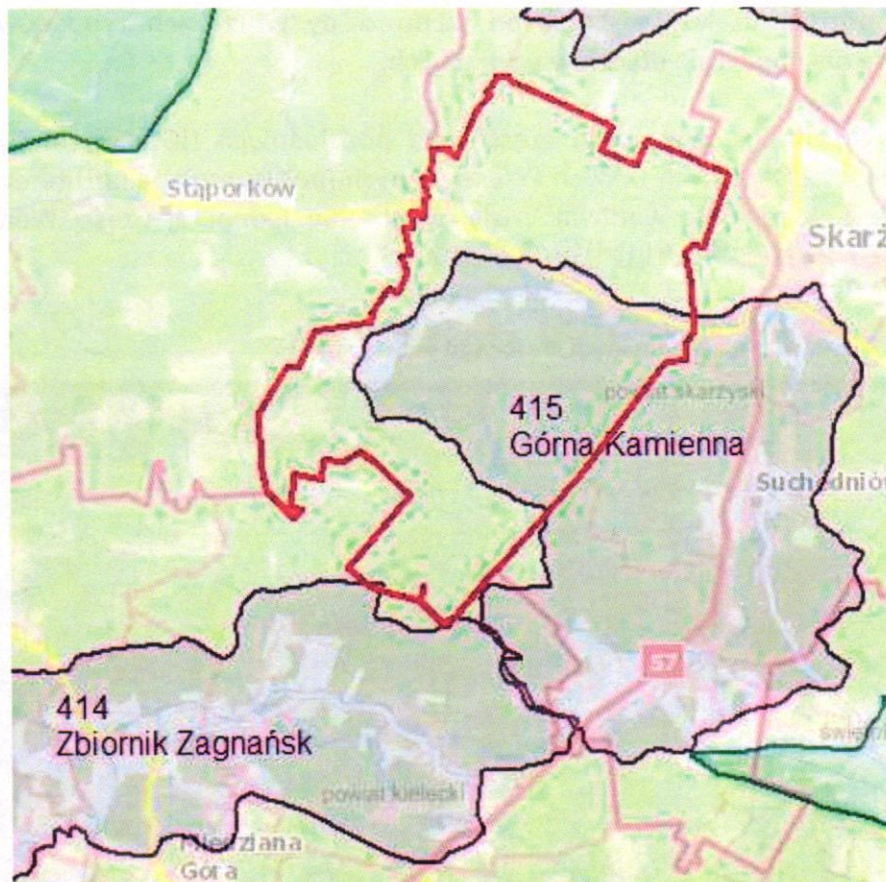
Rysunek 4. Lokalizacja gminy Bliżyn względem Głównych Zbiorników Wód Podziemnych
